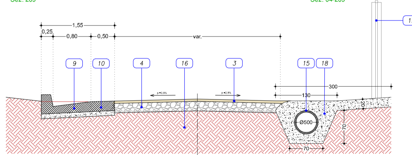
SEZIONI TIPO: SEZIONE CON CAVALCAFOSSO SU UN LATO E CUNETTA E BANCHINA IN C.A.
