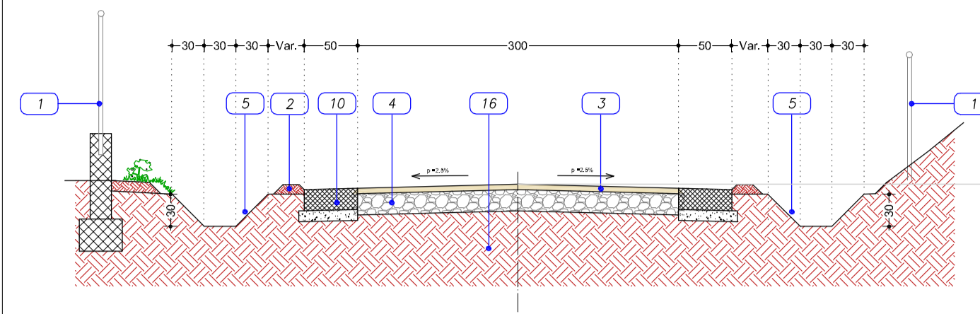
SEZIONI TIPO: SEZIONE CON BANCHINE IN C.A. E CUNETTE IN TERRA SU ENTRAMBI I LATI
