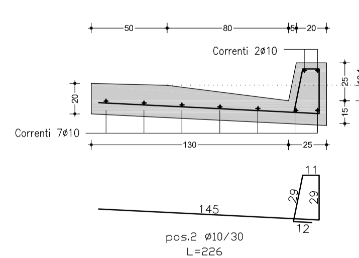
Prospetto delle cunette in c.a.
