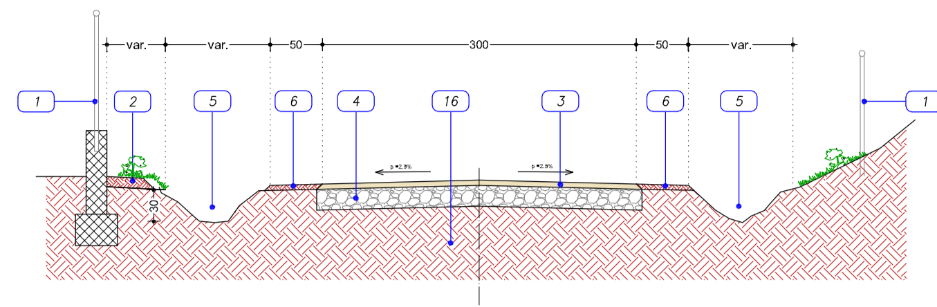
SEZIONI TIPO: SEZIONE CON CUNETTE IN TERRA SU ENTRAMBI I LATI
