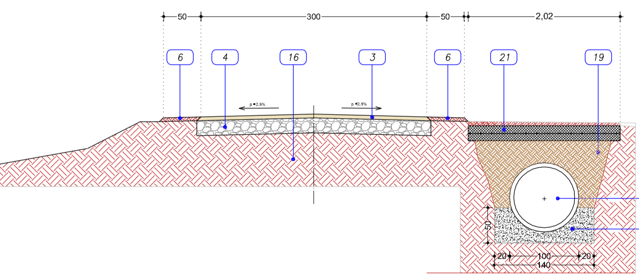
SEZIONI TIPO: SEZIONE CON BANCHINE IN C.A. E CUNETTE IN TERRA SU ENTRAMBI I LATI
