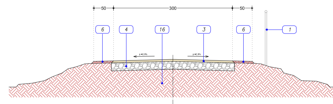
SEZIONI TIPO: SEZIONE CON BANCHINE IN TERRA SU ENTRAMBI I LATI
