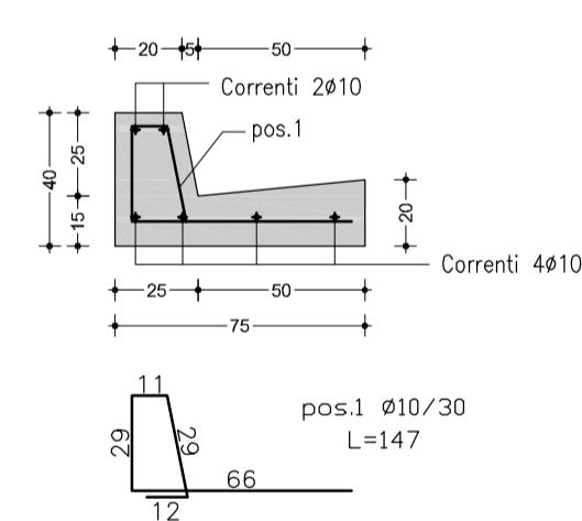
Cunetta b=50 cm (Tipo 1)
