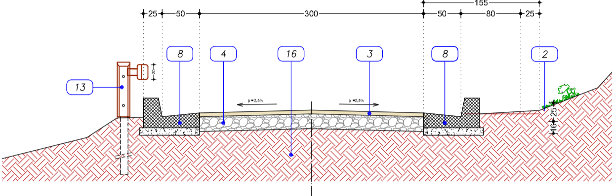
SEZIONI TIPO: SEZIONE CON CUNETTE E BANCHINE IN C.A. SU ENTRAMBI I LATI
