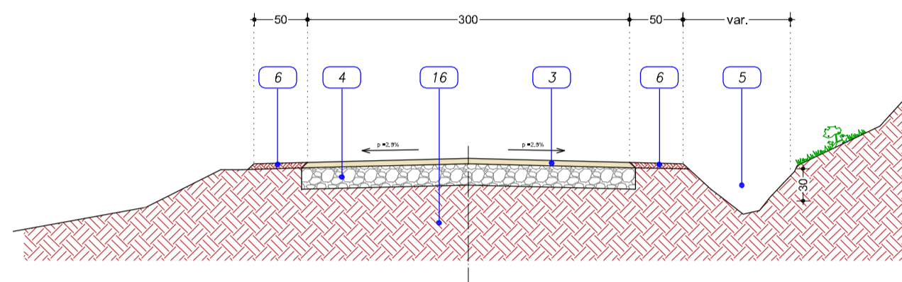
SEZIONI TIPO: SEZIONE CON CUNETTE IN TERRA SU UN SOLO LATO
