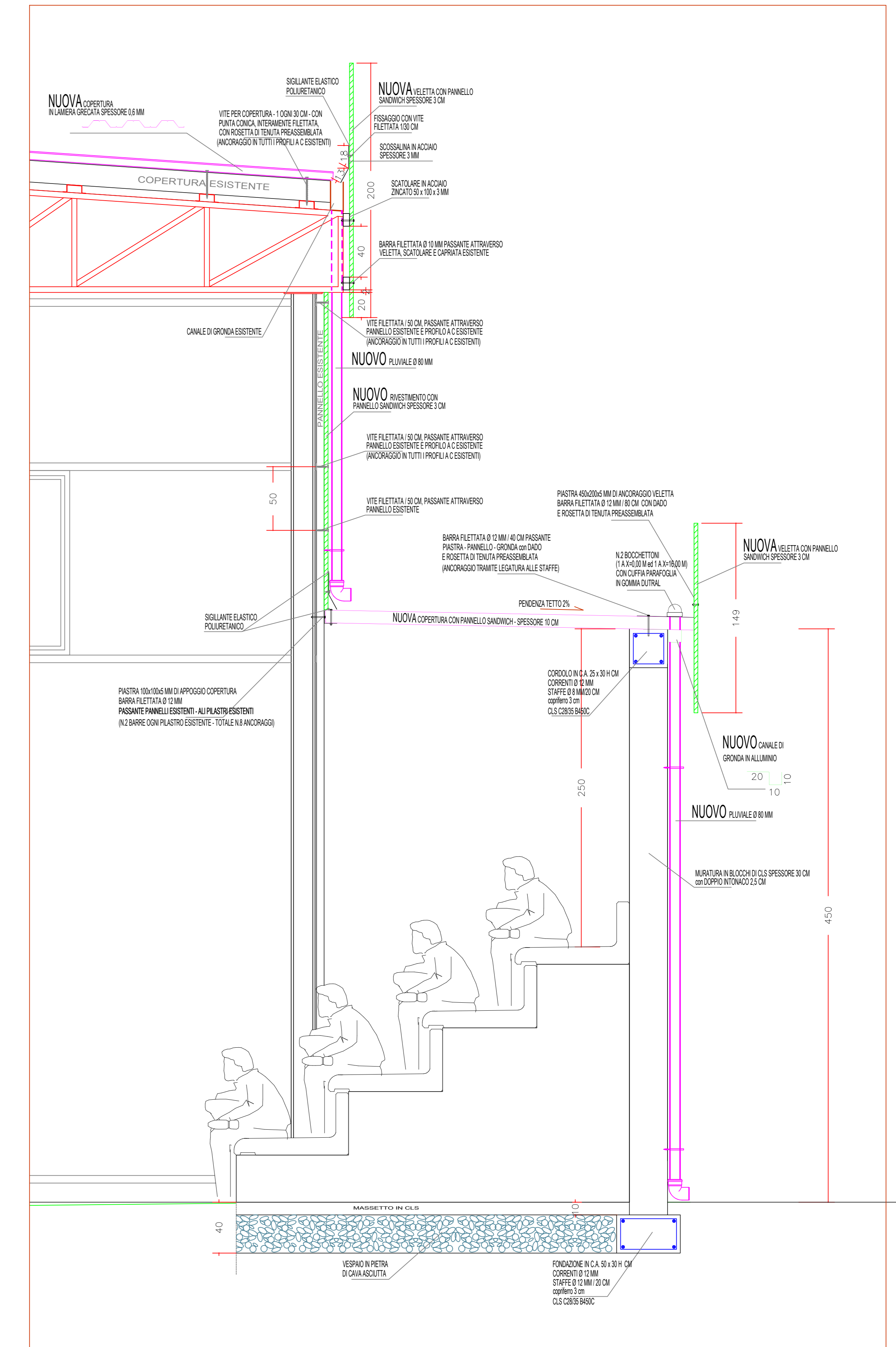
particolare D scala 1:20
