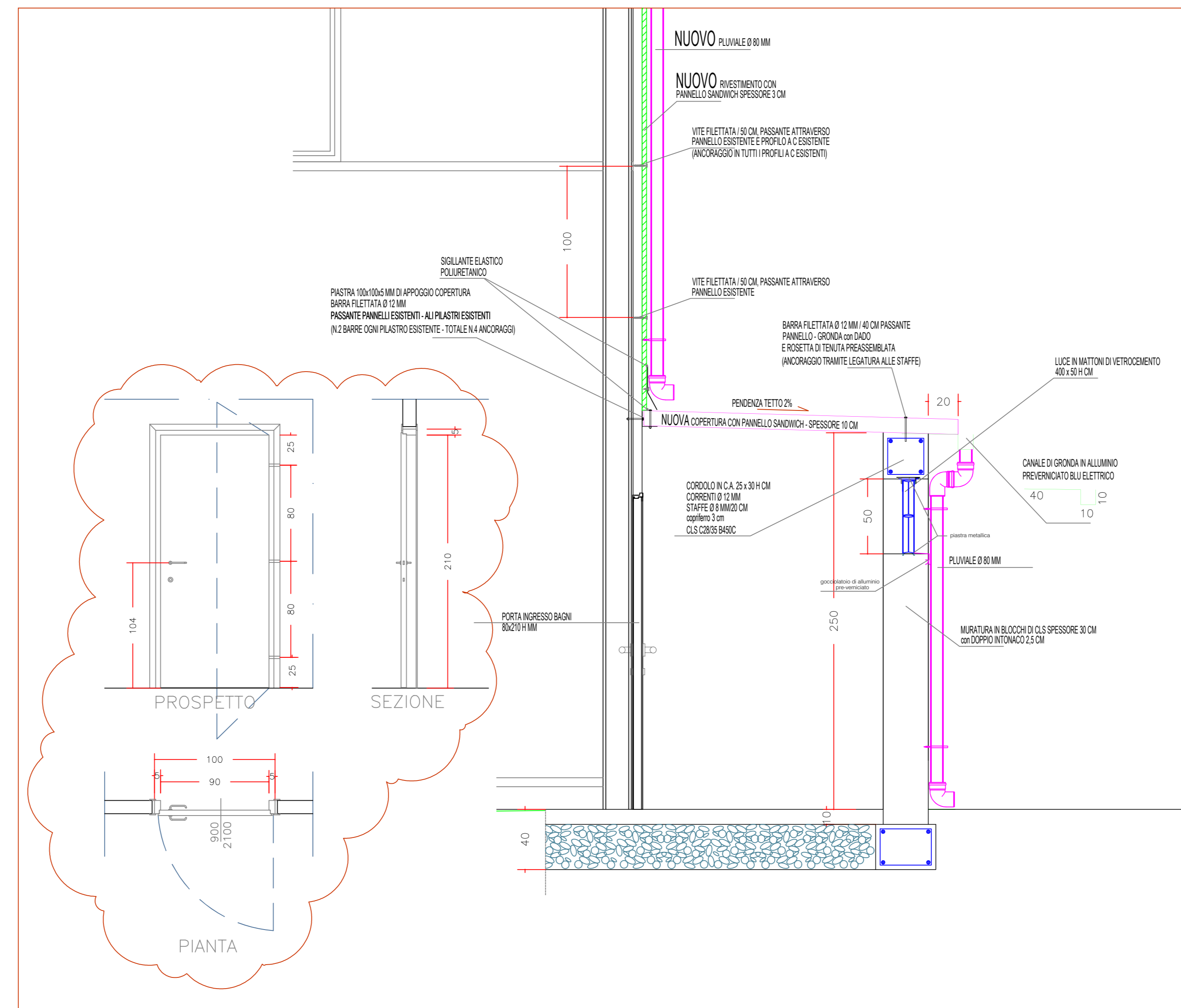
particolare E scala 1:20
